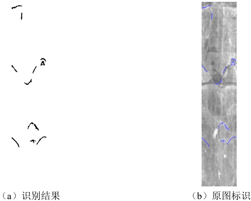
图 4-3-17 图 1-1 识别结果
