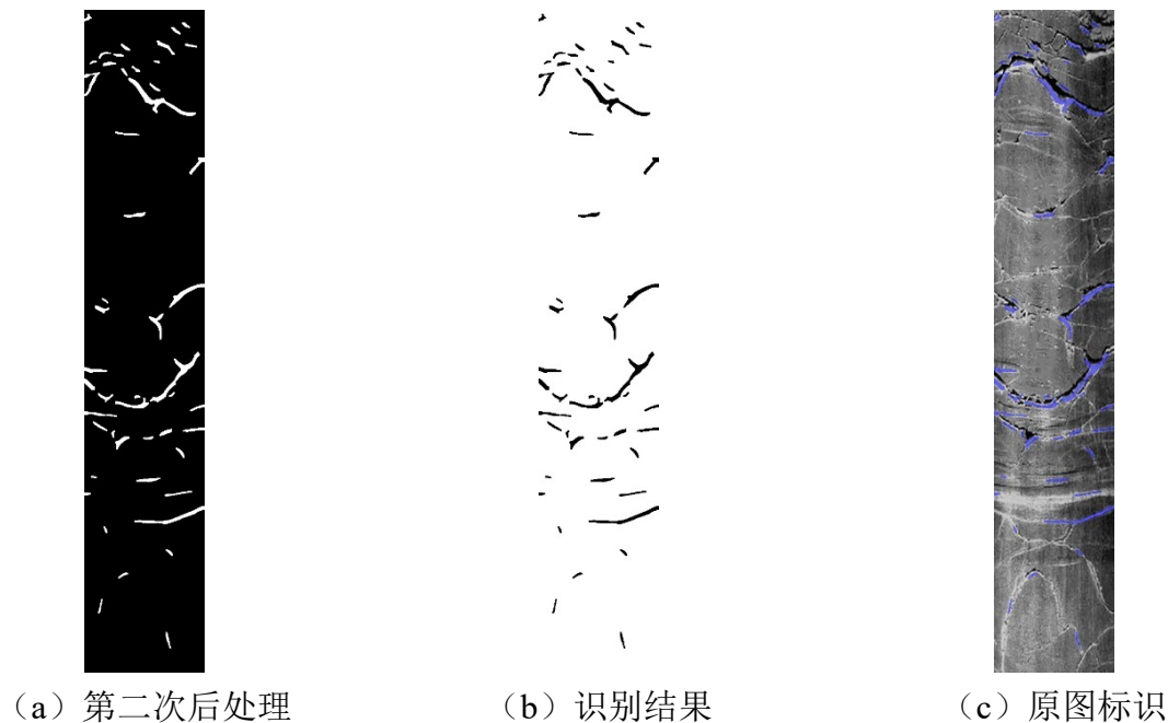
图 4-3-20 图 1-2 识别结果
