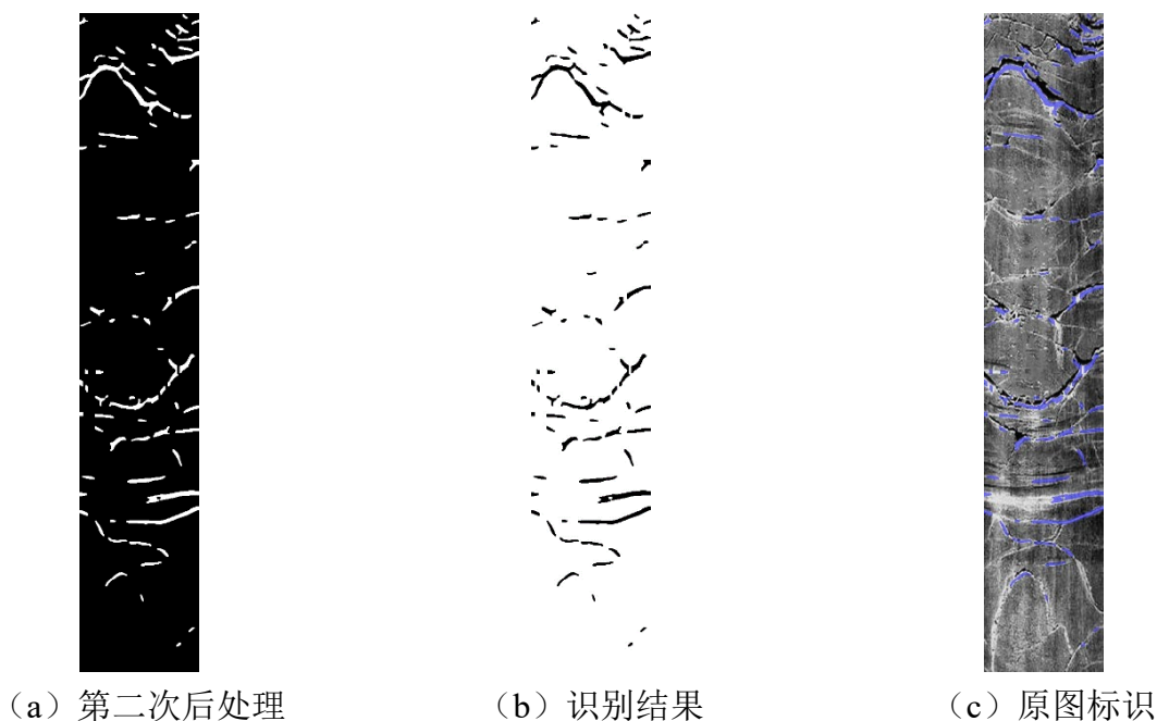
图 4-3-23 图 1-2 识别结果
