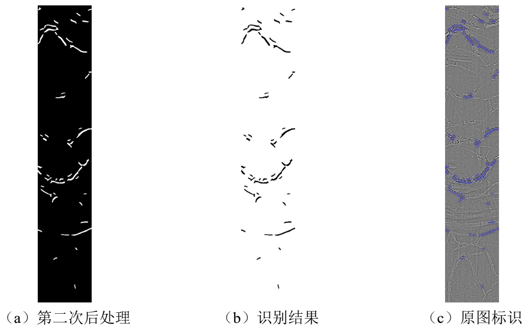
图 4-3-26 图 1-2 识别结果
