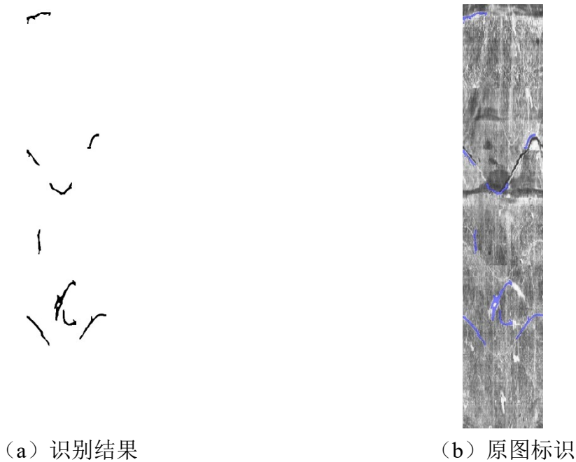
图 4-3-9 图 1-1 识别结果
