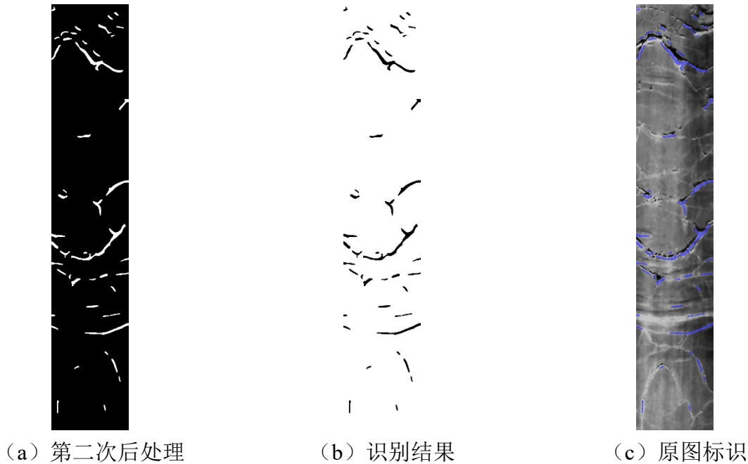
图 4-3-29 图 1-2 识别结果
