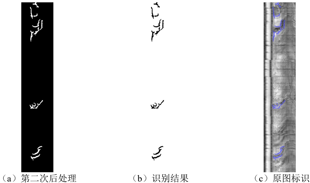
图 4-3-35 图 1-3 识别结果
