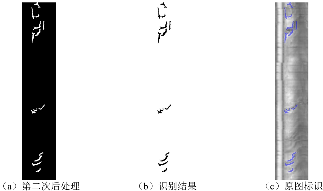
图 4-3-41 图 1-3 识别结果
